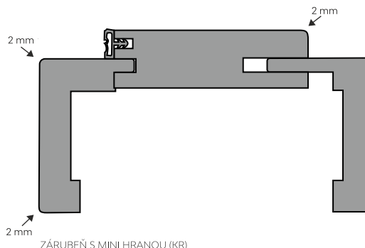
ZÁRUBĚN S MINI HRANOU (KR)
